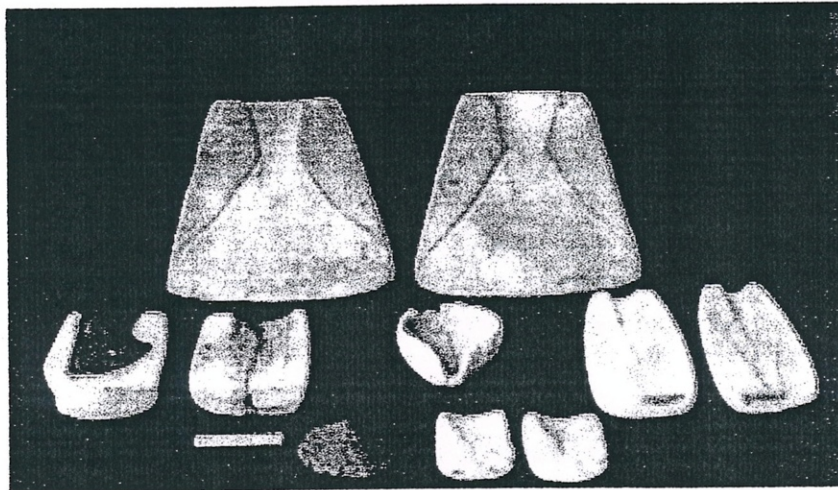
แม่พิมพ์ทำด้วยหินทราย และเบ้าหลอมทำด้วยดินเผา เป็นอุปกรณ์ในการหล่อวัตถุสำริด พบที่แหล่งโบราณคดีวัฒนธรรมบ้านเชียง ในภาคตะวันออกเฉียงเหนือของประเทศไทย
